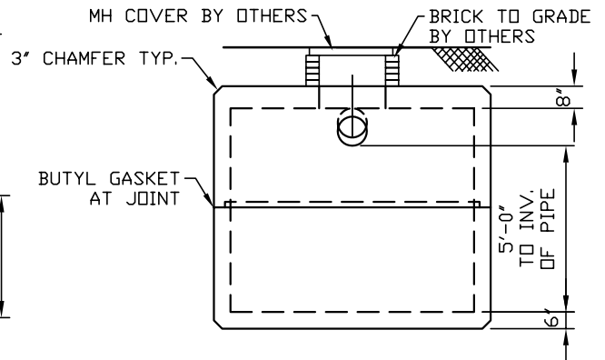
ELEVATION A-A
